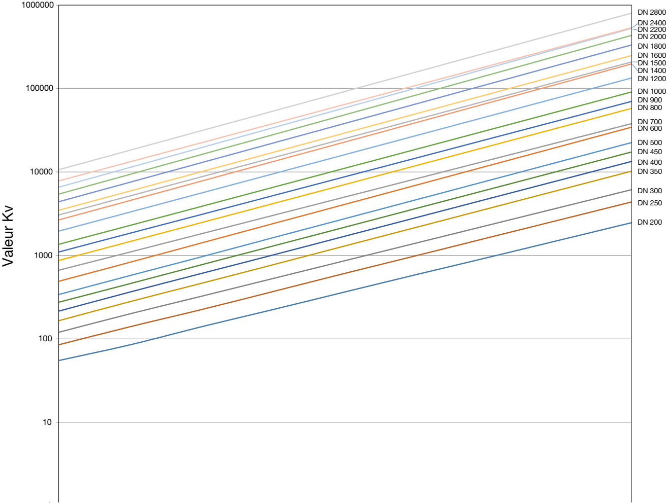
Valeurs KV pour vannes papillon DN 200 - 2800
